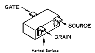
2SK208Y(JY) (Q6074)
