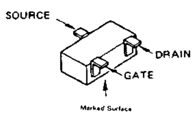
2SK302GR(TG) (Q6069) 2SK302Y(TY) (Q6056, Q6070)
