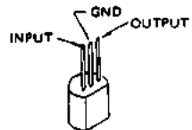
μPC78L05J (Q1027)
