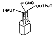
MFC78L05J (Q1027)
