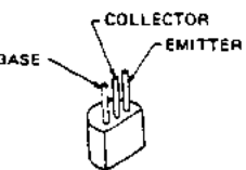
2SD667C (Q3027)
