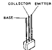
BA1A4M (Q7203)
