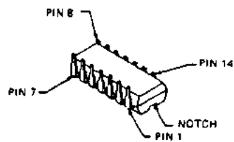
MC14011BCP (Q1030)
