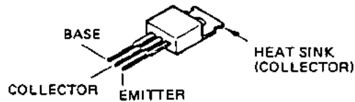
2SB5950 (Q7607)
