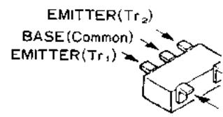
Marked Sur FMC3(T) (Q6106)
