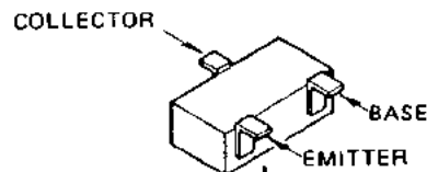
Marked Surface 2SC2712GR(LG) (Q3002, Q3002, Q3012, Q3012, Q3035, Q3035, Q3054, Q3054) FA1A4P(L34) (Q3018, Q3021, Q3022, Q3026, Q3033, Q3037, Q3038, Q3046, Q3058, Q3060, Q3063, Q3068, Q3070, Q3071, Q3078, Q3078) FA1F4N(L35) (Q3067) FN1A4P(M34) (Q3047, Q3059, Q3061, Q3084)
